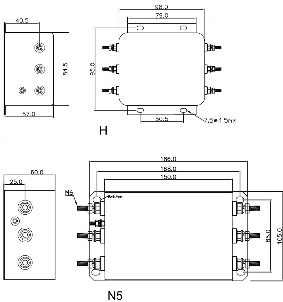
外形尺寸 Outline Dimensions(mm)
